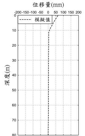
(b) FH-23 地中變形模擬成果
