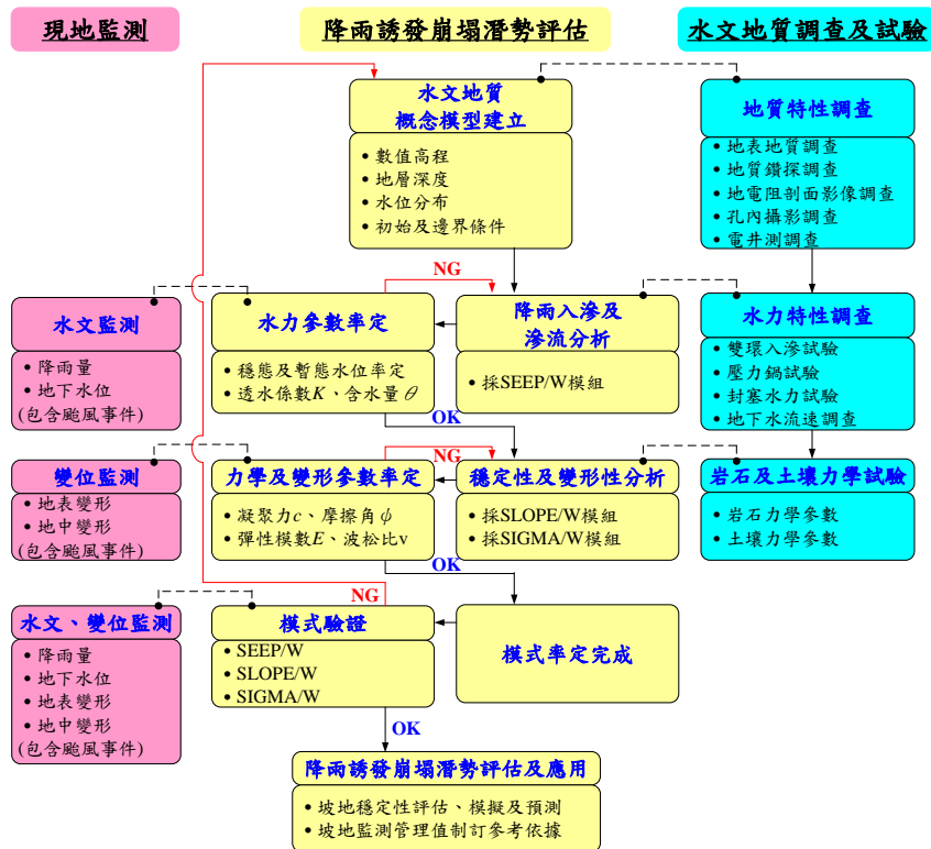
圖 5 降雨誘發崩塌潛勢評估流程圖
