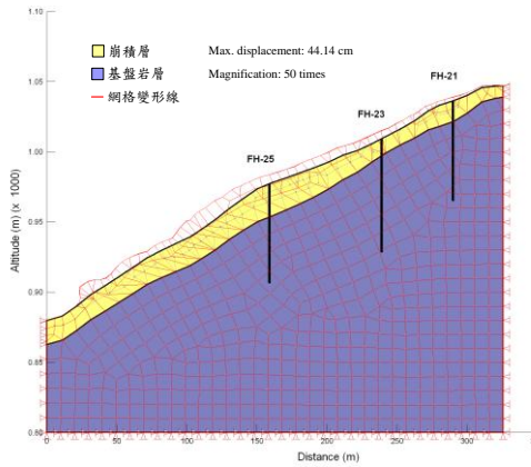
(a) 網格變形示意圖
