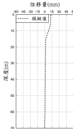
(a) FH-21 地中變形模擬成果
