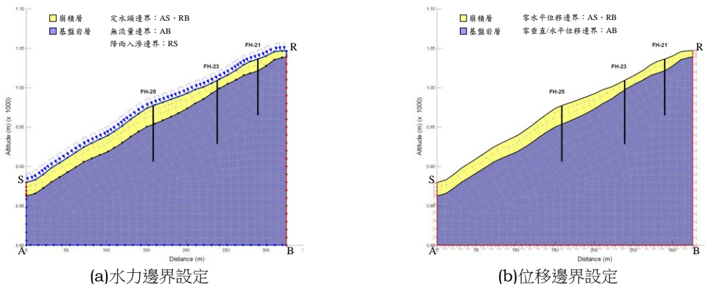
圖 6 吉露調查範圍水文地質概念模型與邊界條件
